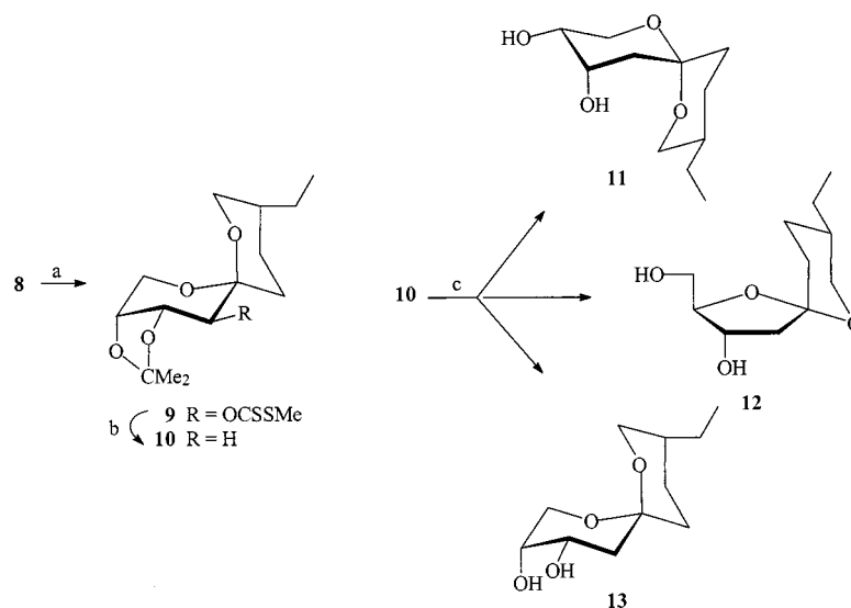
Scheme 5. Deisopropylidenation of 10 : a: NaH/THF/imidazole/ \text{CS}_2 /MeI; b: \text{H}_3\text{PO}_4 /dioxane/ \text{H}_2\text{O} / \text{Et}_3\text{N} /AIBN; c: AcOH/ \text{H}_2\text{O} /40 °C/45 min
